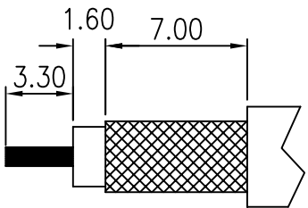
CABLE STRIPPING DIM.
