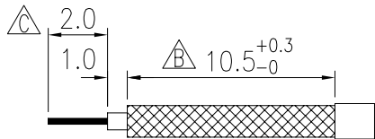
CABLE STRIPPING DIM.
