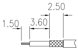
CABLE STRIPPING DIM.
