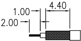
CABLE STRIPPING DIM.
