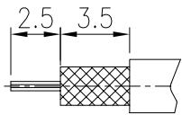
CABLE STRIPPING DIM.
