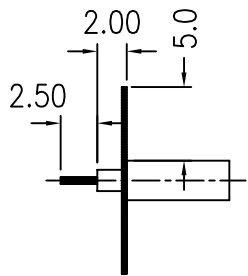
CABLE STRIPPING DIM.
