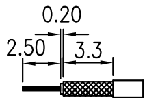
CABLE STRIPPING DIM.
