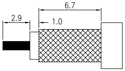
CABLE STRIPPING DIM.
