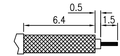
CABLE STRIPPING DIM.
