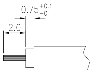
CABLE STRIPPING DIM.
