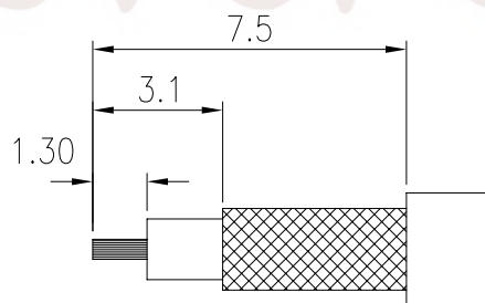
CABLE STRIPPING DIM.
