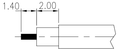
CABLE STRIPPING DIM.
