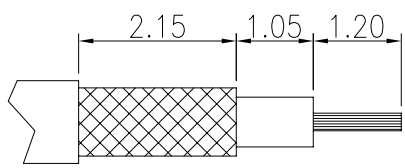
CABLE STRIPPING DIM.
